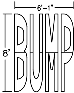
8' BUMP Legend 90 mil HotTape Item # HT894800 125 mil HotTape Item # HT894108
